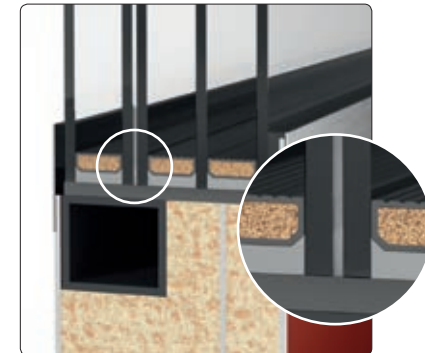
Angriffhemmende Verglasung der Klasse P5A gemäß DIN EN 356
