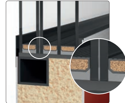
Angriffhemmende Verglasung der Klasse P4A gemäß DIN EN 356
