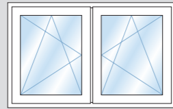
Zweiflügelige Fenster | Fenstertüren mit festem Setzposten
