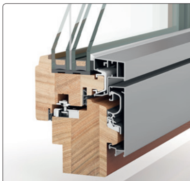
PaXoptima78 flächenbündig**
