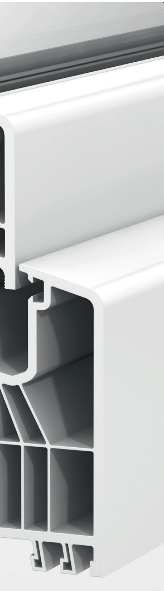
Der solide doppelwandige Mittelsteg erschwert das Einstechen mit einem Hebelwerkzeug und schützt auf diese Weise den Beschlag.
