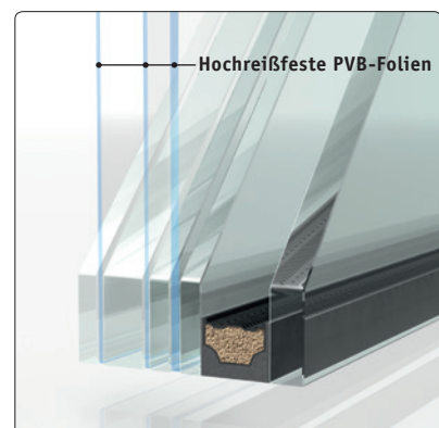
Durchbruchhemmende Verglasung der Klasse P6B nach DIN EN 356
